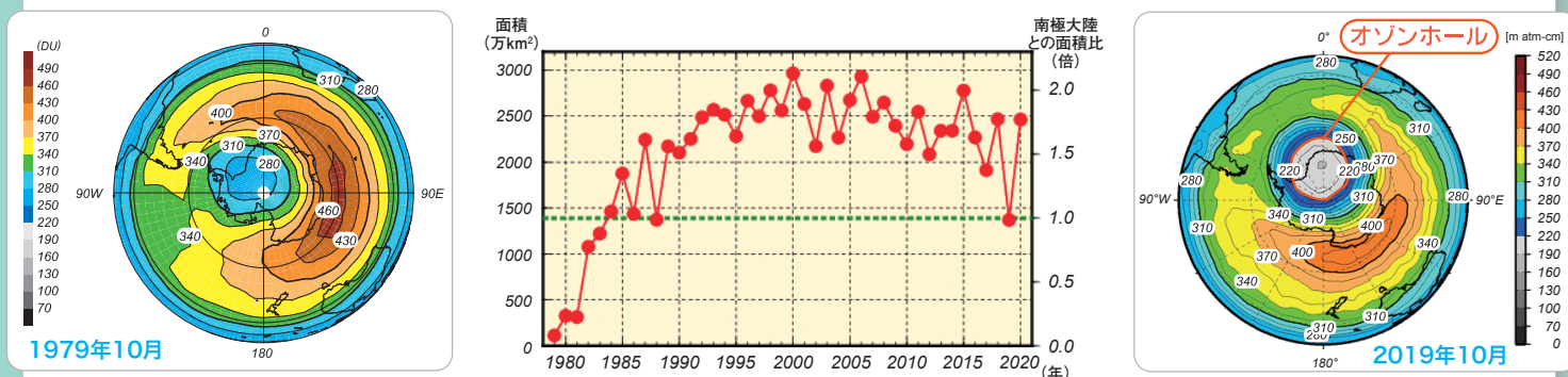
オゾンホールの年最大面積の経年変化（中央折れ線グラフ）と南半球の10月の月平均オゾン量の分布（左右図） データ提供：気象庁
