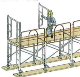
・足場の手すり先行工法の採用
